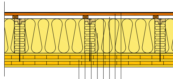
Horizontalsnitt, ISOVER PLUS + på KL-trä
